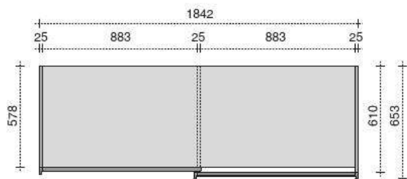
Armadio bloccato con 2 ante da "90" Fixed body wardrobe with 2 doors "90"
