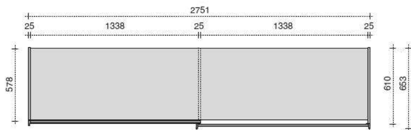
Armadio bloccato con 2 ante da "135" Fixed body wardrobe with 2 doors "135"
