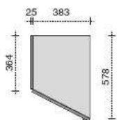
Elemento Terminale Obliquo SX con 1 ante battente LH Oblique end element with 1 door
