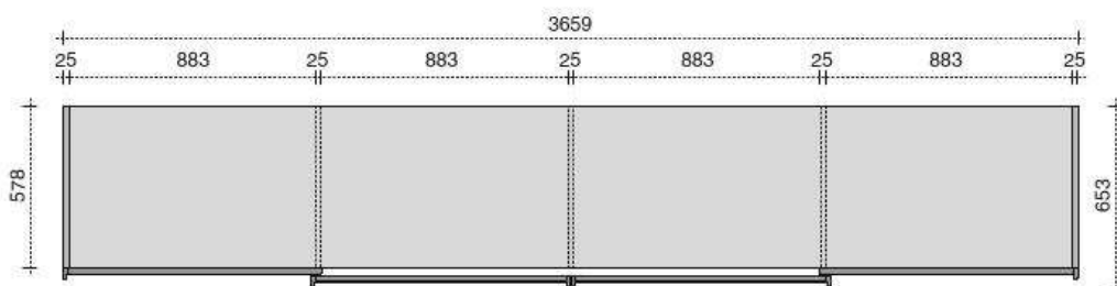
Armadio bloccato con 4 ante da "90" Fixed body wardrobe with 4 doors "90"
