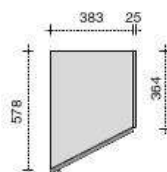
Elemento Terminale Obliquo DX con 1 ante battente RH Oblique end element with 1 door
