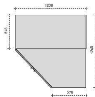
Angolo Spogliatoio DX Corner Dressing Cabinet
