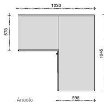
Angolo con 2 ante battenti Corner with 2 doors
