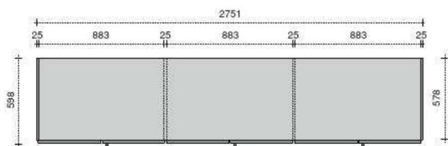
Armadio bloccato con 6 ante battenti Fixed body wardrobe with 6 doors
