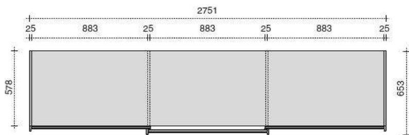
Armadio bloccato con 3 ante da "90" Fixed body wardrobe with 3 doors "90"
